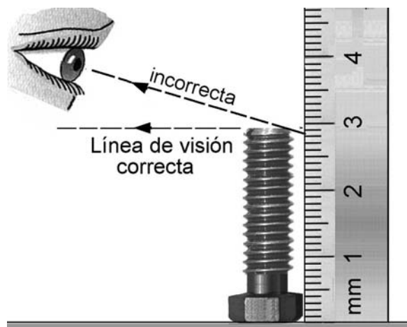
Fig. 4: Un error de paralaje
